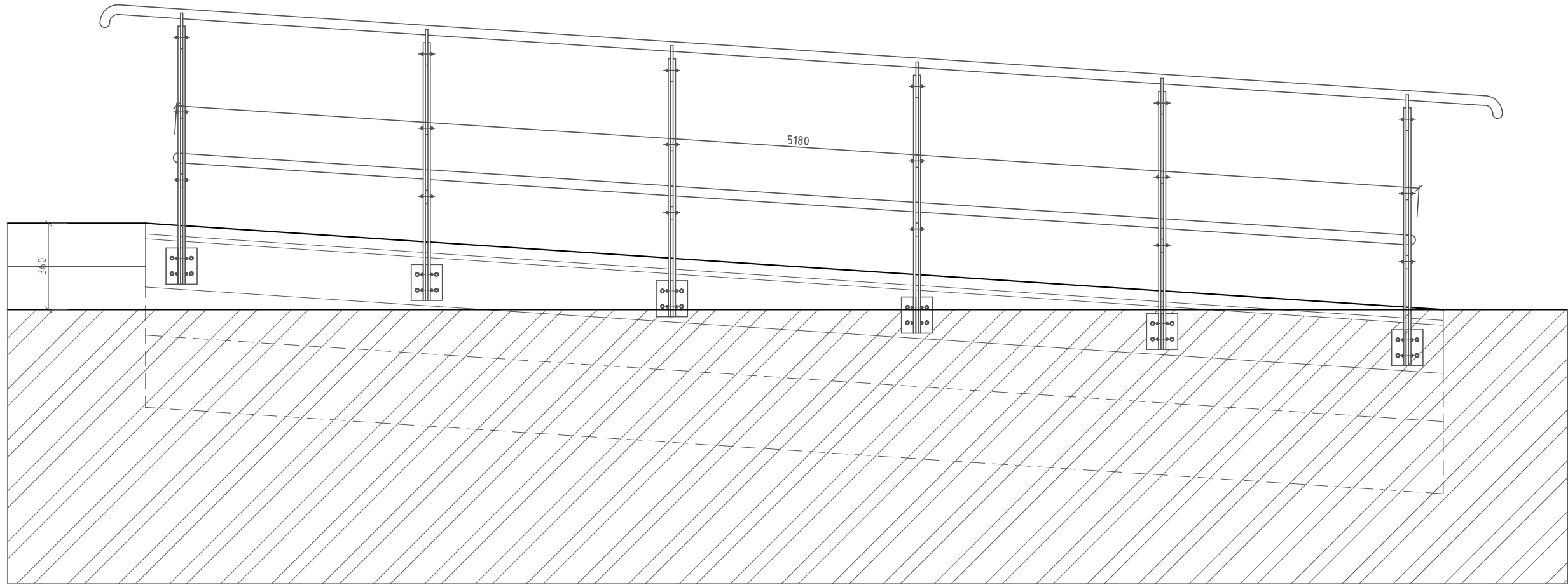
POHL'AD M= 1:20
