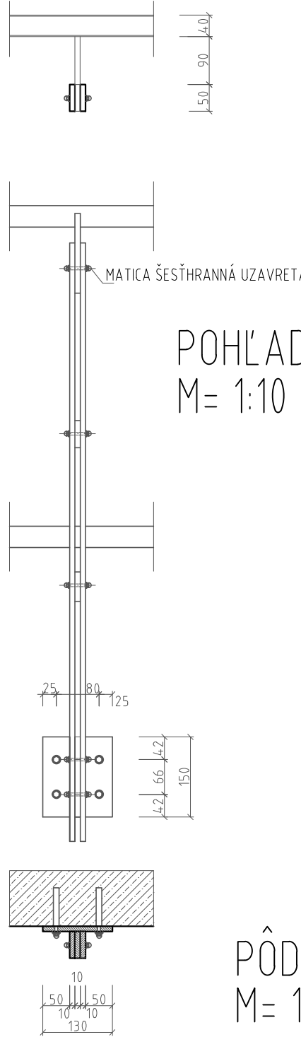
PÔDORYS M= 1:10
